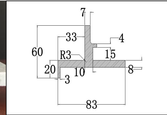
Door frames
